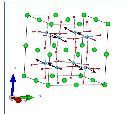
Ti_Au_1
