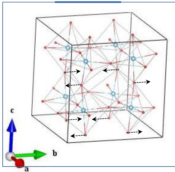
O2_B3u_1
