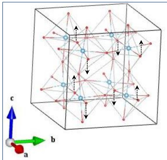
O1_B2u_2
