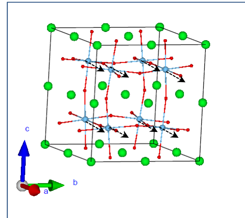
Ti_B 3u _1
