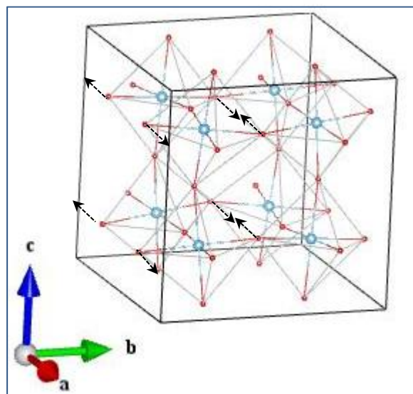
O3_Ag_2
