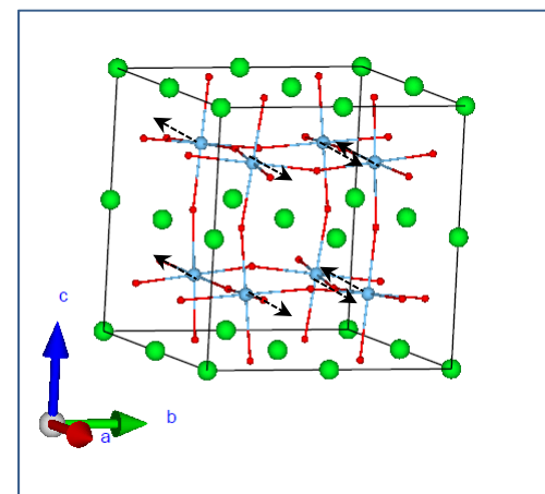
Ti_B2u_1
