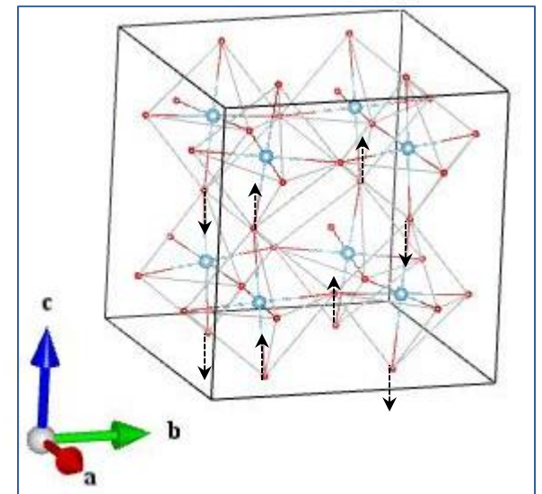
O1_Au
