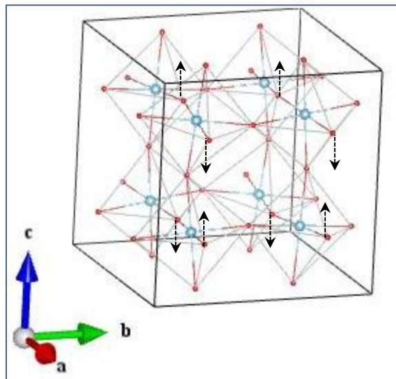
O1_Ag_2
