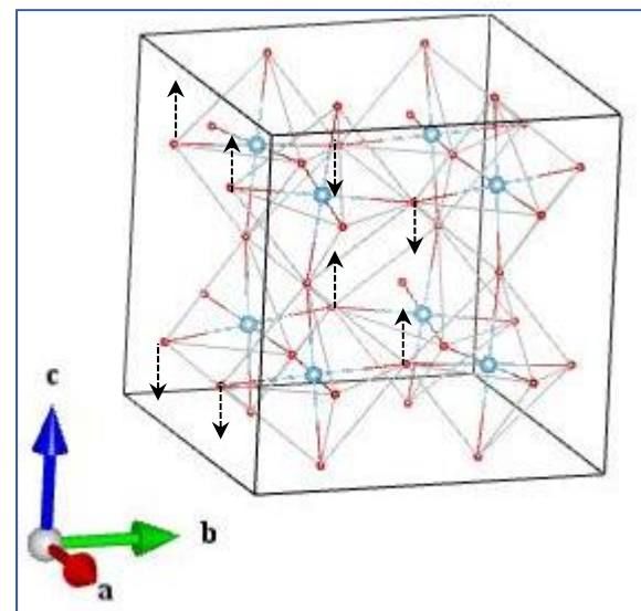
O3_Ag_1
