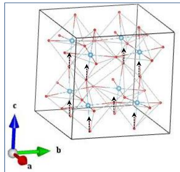
O2_B1u
