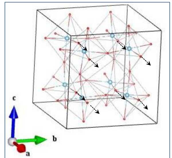
O1_B3u
