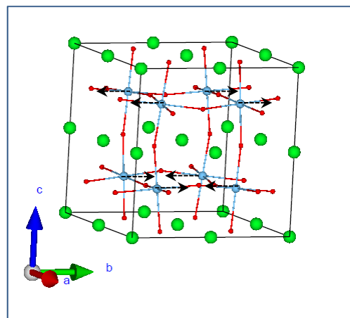
T B1u_2
