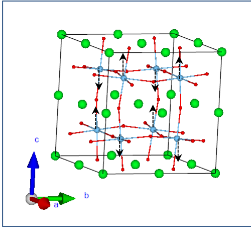
Ti_B 3u _3
