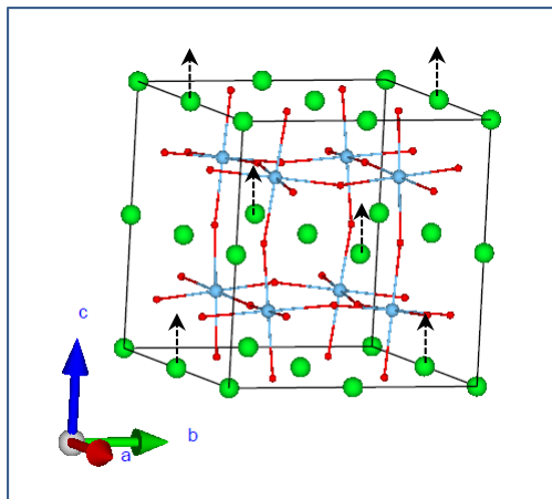
Sr_2_B1u
