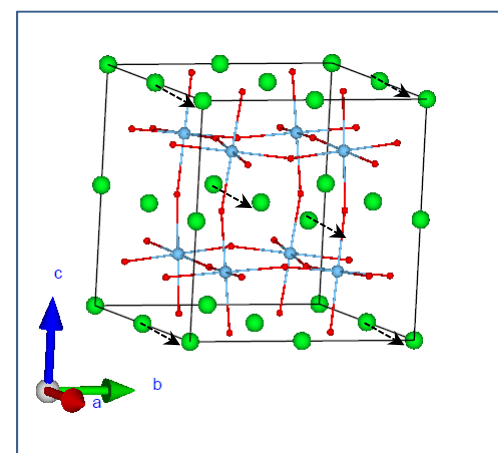
Sr_2_B3u
