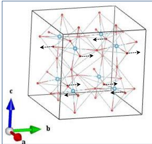
O1_B3g_1
