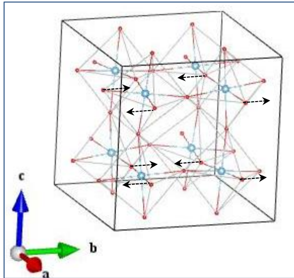
O1_Ag_1
