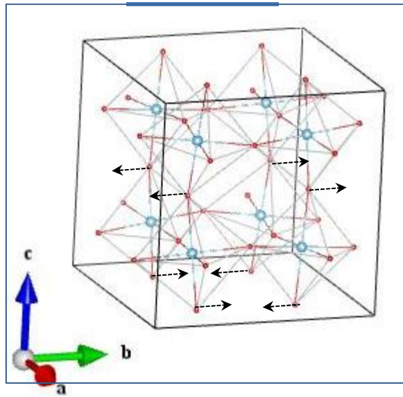
O2_Ag_1
