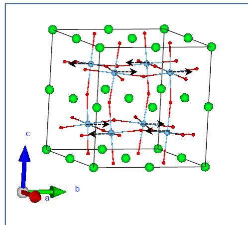
T_Au_2
