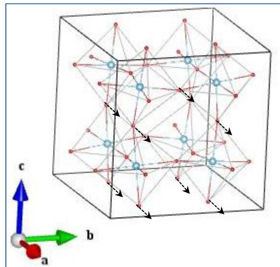
O2_B3u_2
