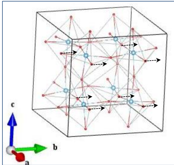
O1_B2u_1
