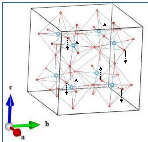
O1_B3g_2
