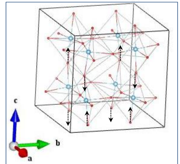
O2_B2g
