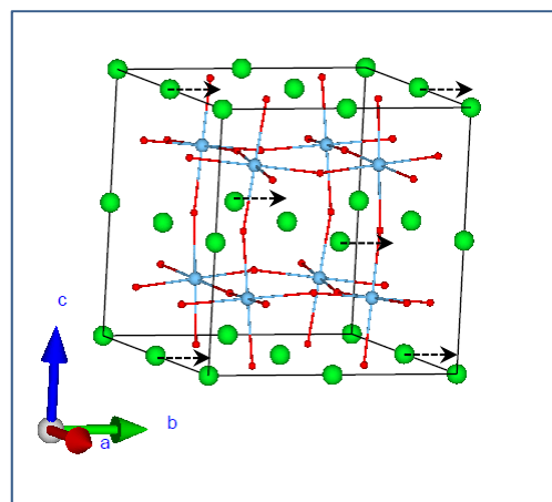
Sr_2_B2u
