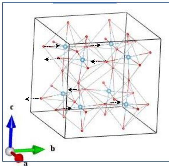
O3_Au
