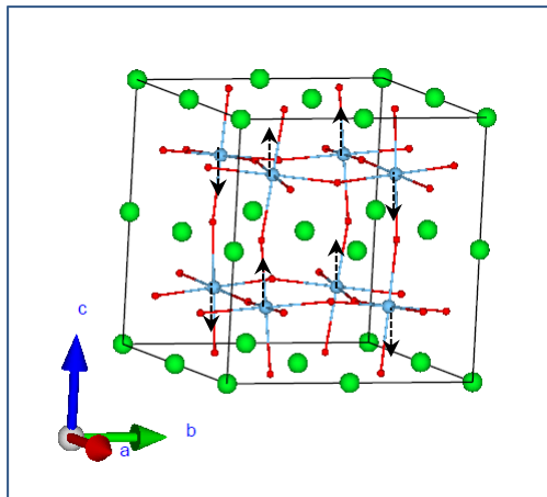
Ti_Au_3
