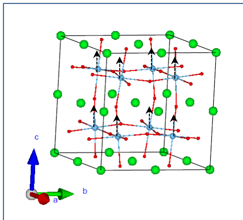
Ti B1u_3
