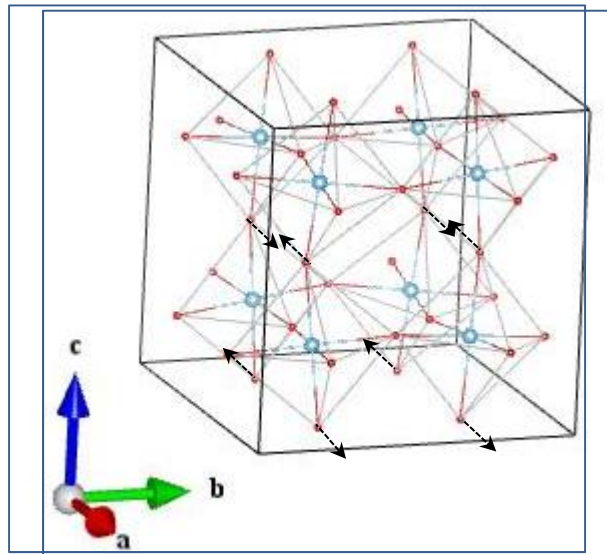
O2_Ag_2
