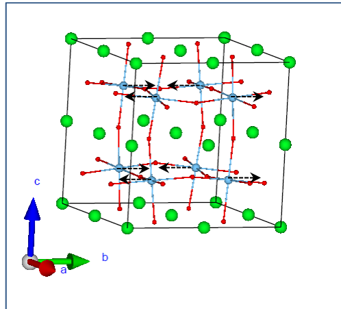
T_B 3u _2
