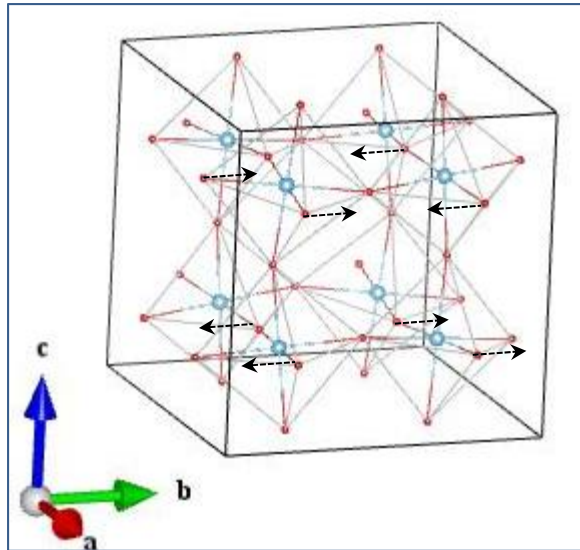
O1_B1u_1
