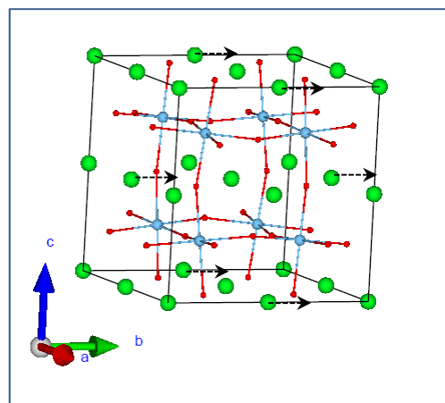
Sr_4_B2u
