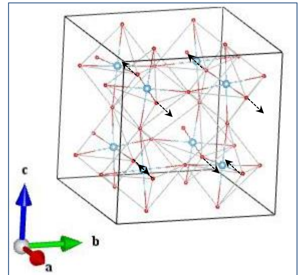
O1_B2g
