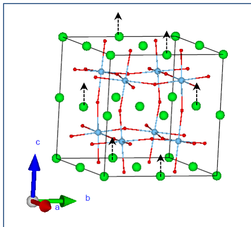
Sr_4_B1u
