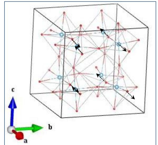
O1_B1g
