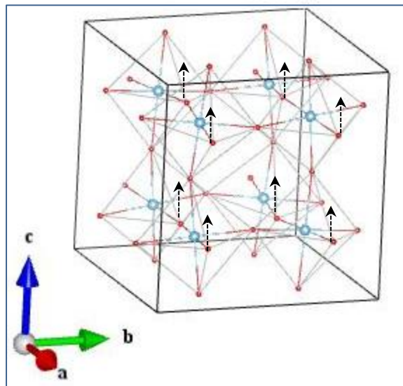
O1_B1u_2
