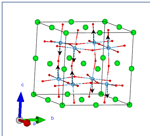
Ti_B2u_3
