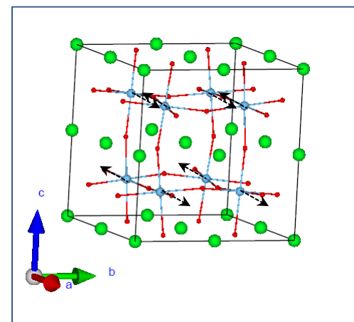
Ti B1u_1
