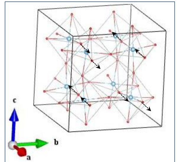
O1_Au
