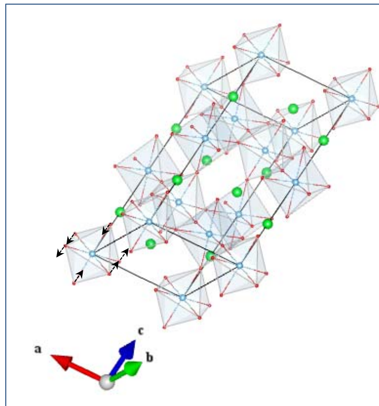
O_A 2g (1_2)
