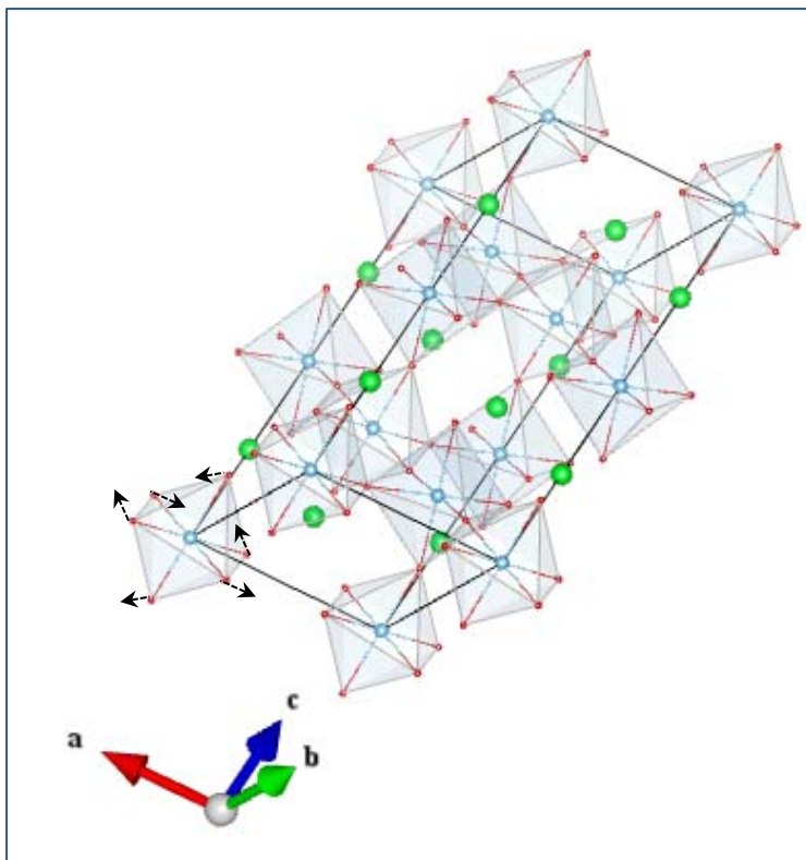
O_Eu(2_1)
