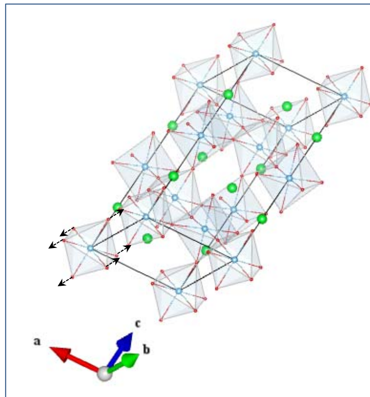
O_Eg(1_2)
