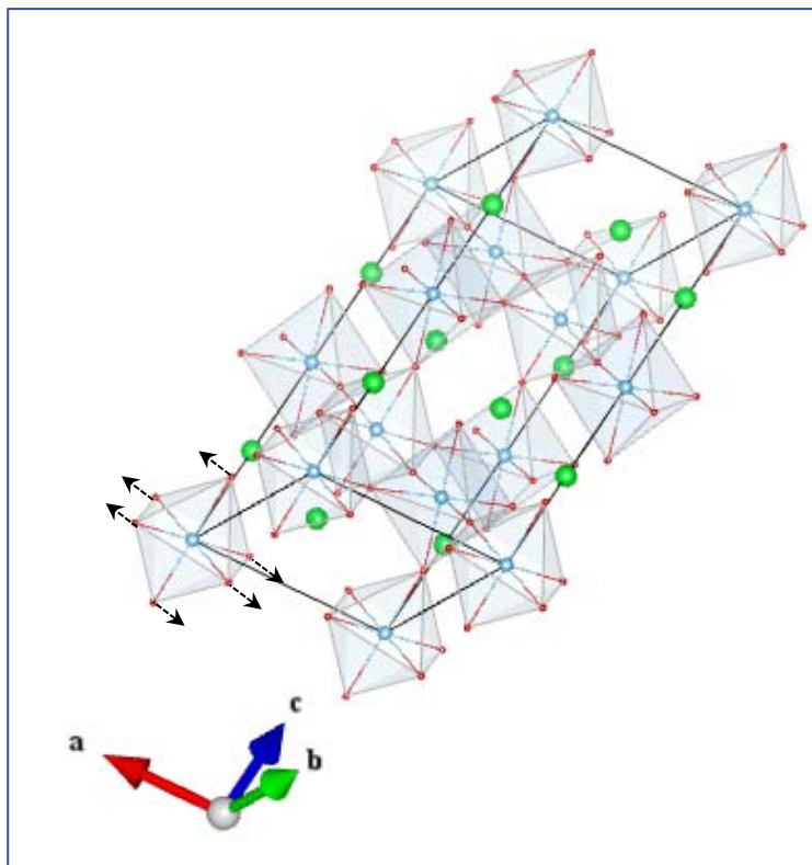
O_Eg(1_1)
