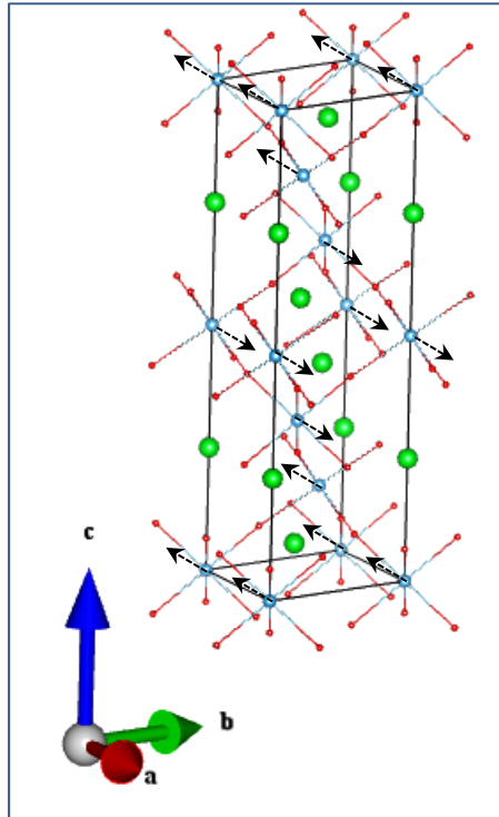
Ti_Eu(2_1)
