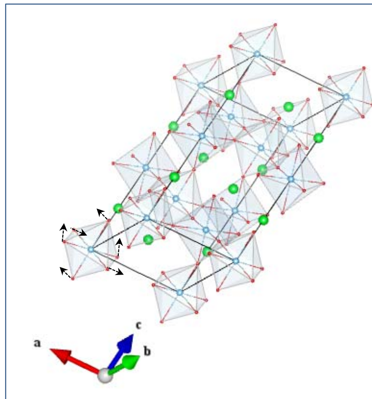
O_Eu(2_2)
