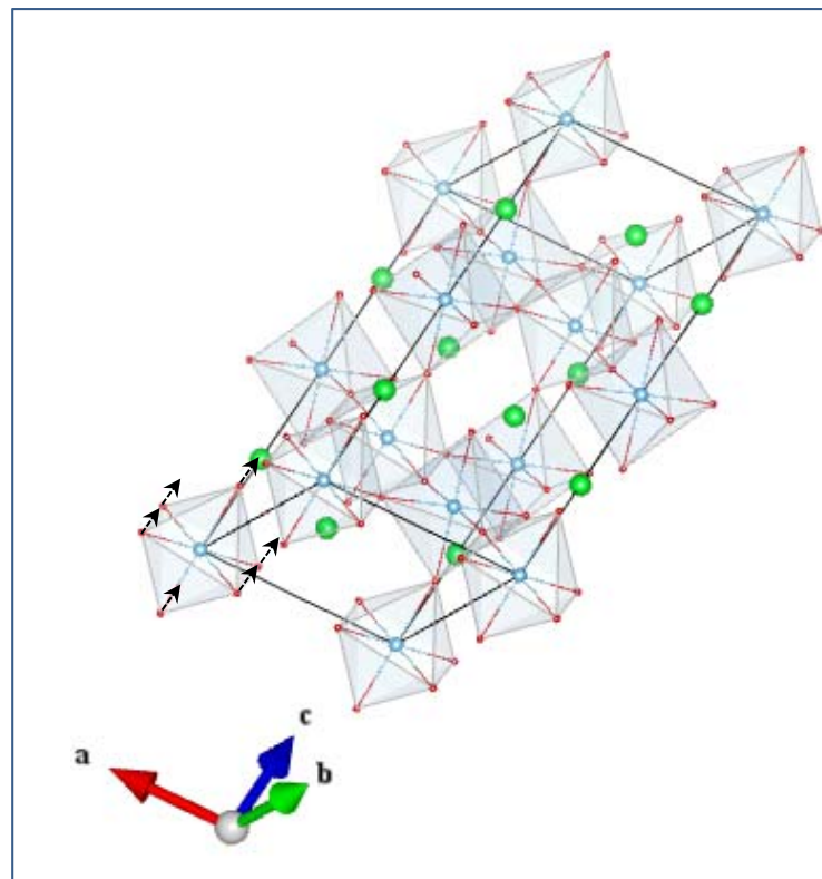
O_A 2u (1_2)
