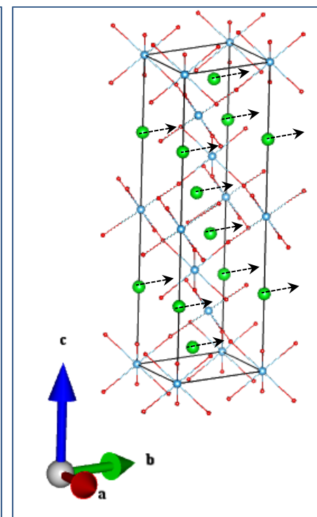
Sr_Eu (1_2)
