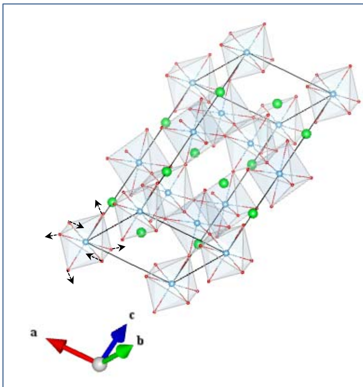
O_A 2g (1_1)
