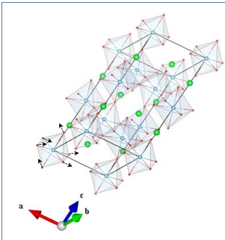
O_A 2u (1_1)
