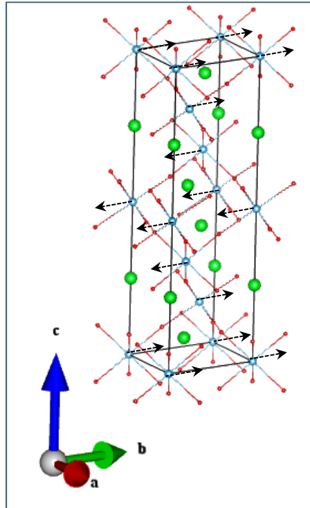
Ti_Eu(2_2)
