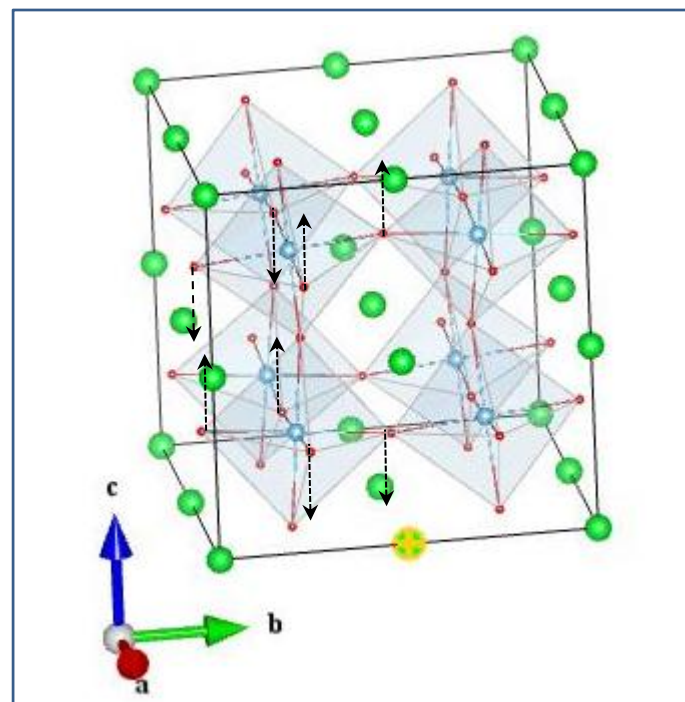
O1_B 1g (1_2)
