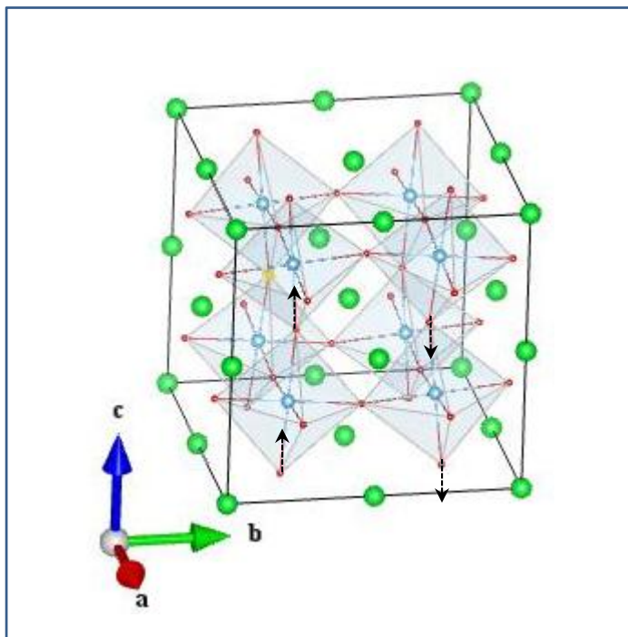
O2_B 1u (1)
