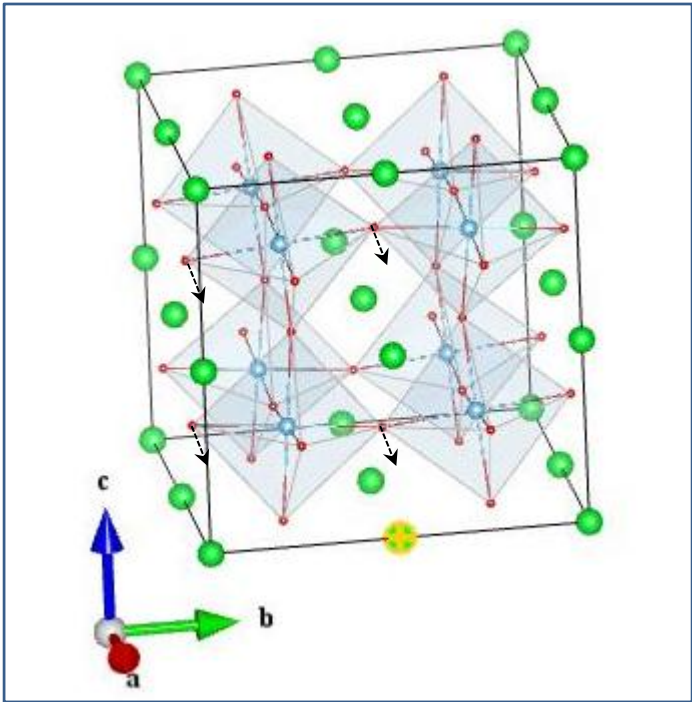
O1_Eu(2_1)
