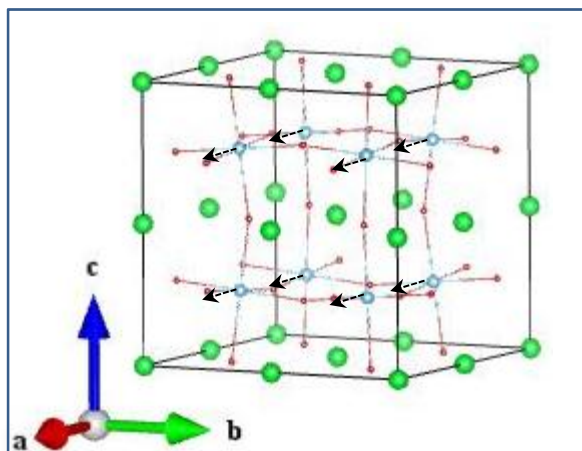
Ti_Eu (1_1)
