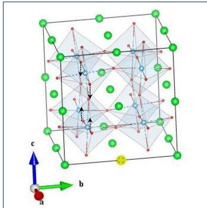
O1_Eu(1_2)
