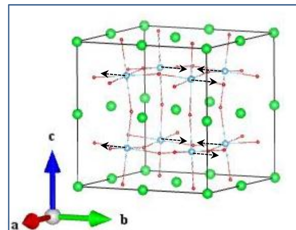
Ti_Eu (2_1)
