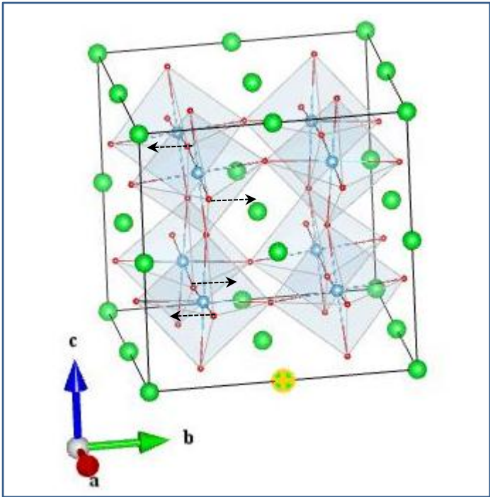
O1_Eg(1_1)
