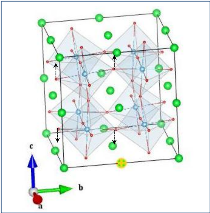
O1_Eu(1_1)
