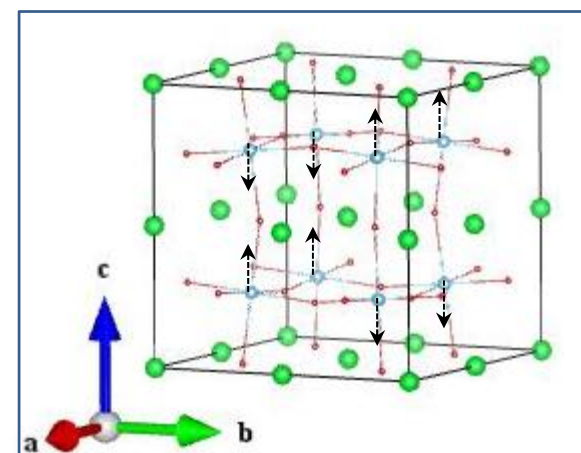
Ti_Eu (3_2)
