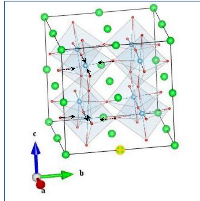
O1_B 2g (1)
