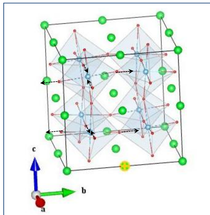
O1_A 2g (1)
