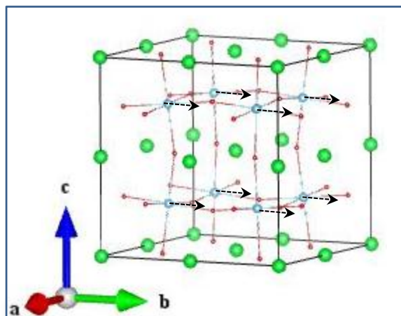
Ti_Eu (1_2)
