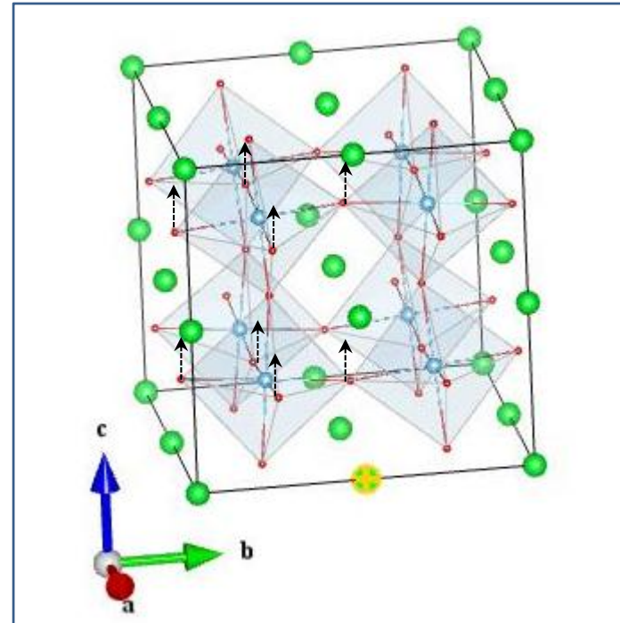
O1_A2u(1_2)
