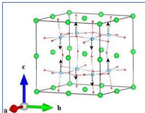
Ti_B 1u (1_2)
