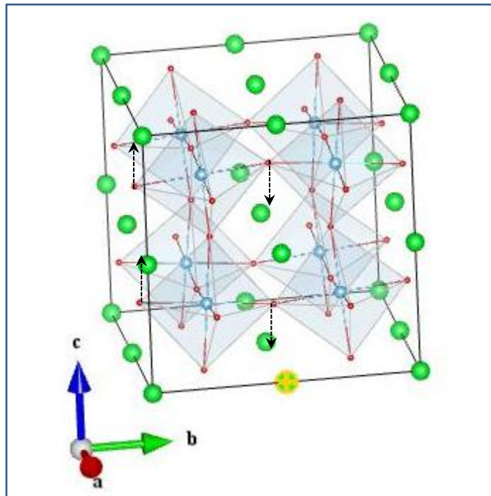
O1_Eg(3_2)
