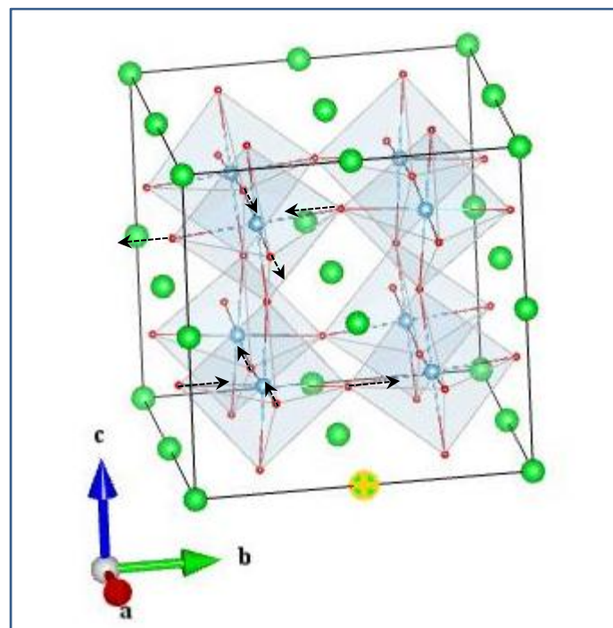
O1_B 1u (1)
