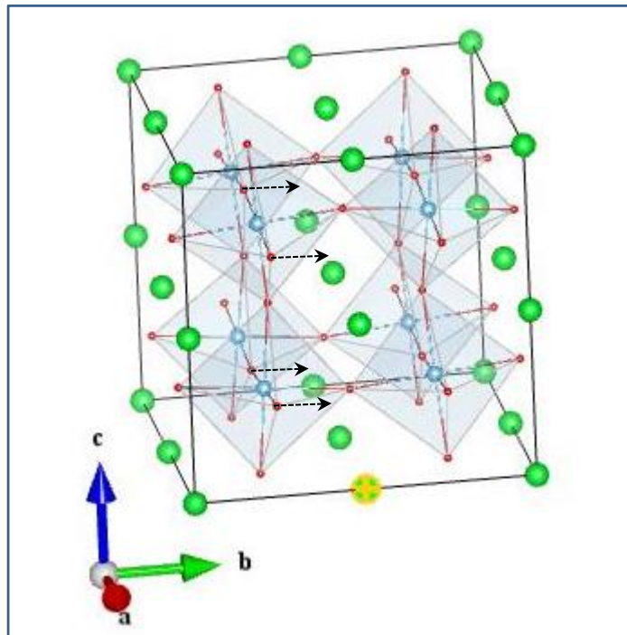
O1_Eu(2_2)
