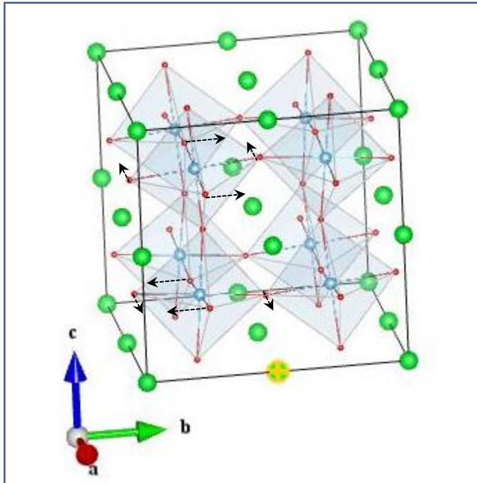
O1_A2u(1_1)
