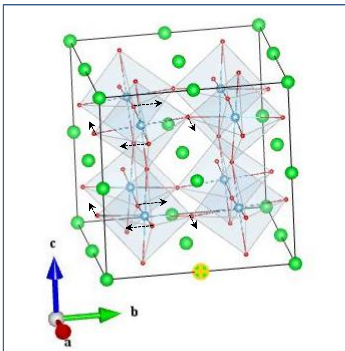
O1_B 1g (1_1)
