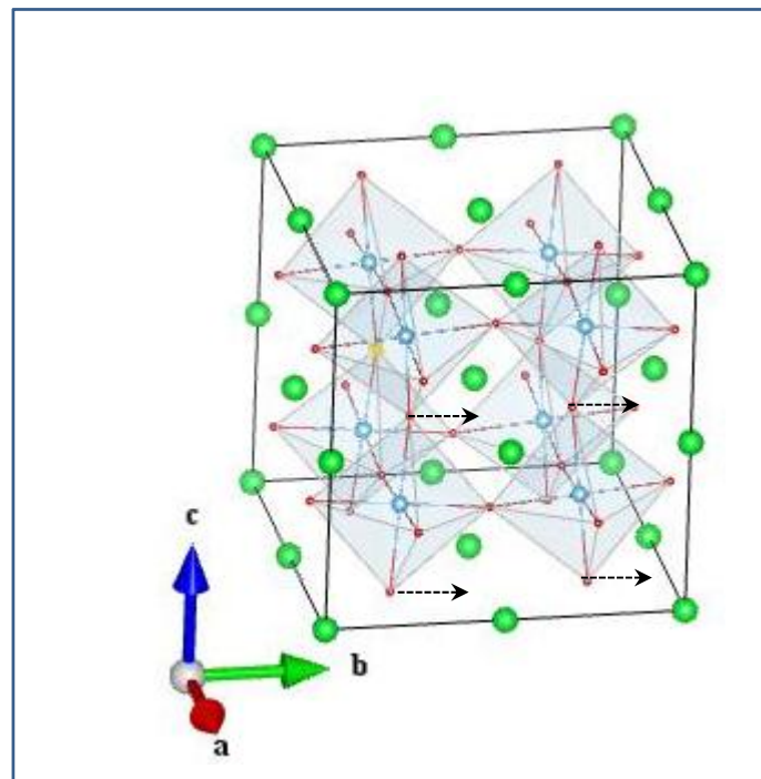
O2_Eu(2_2)
