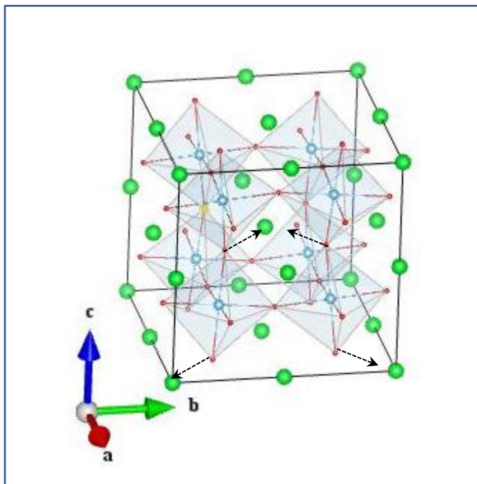
O2_A1g(1_1)
