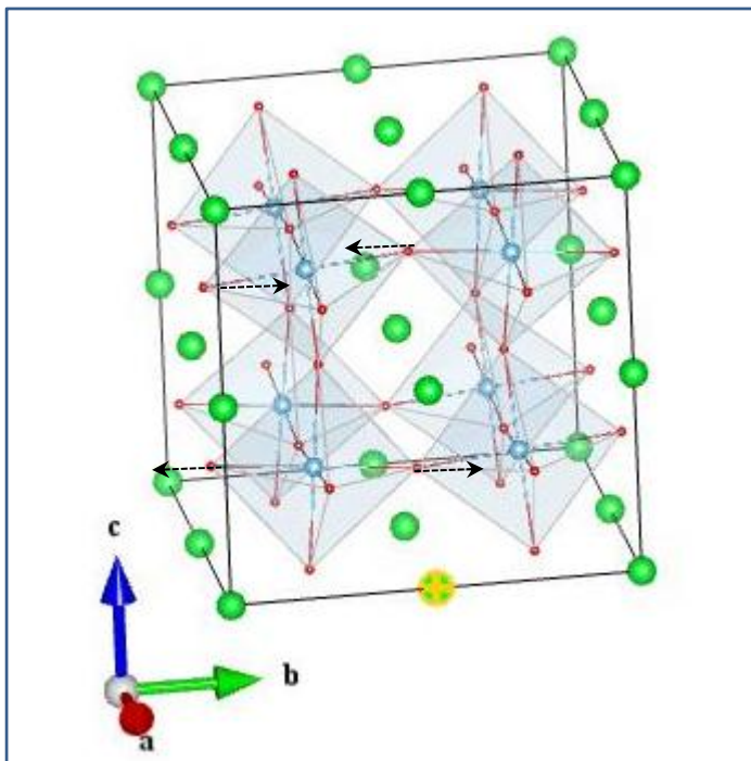
O1_Eg(2_1)
