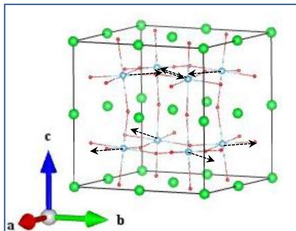
Ti_A 2u (1_1)
