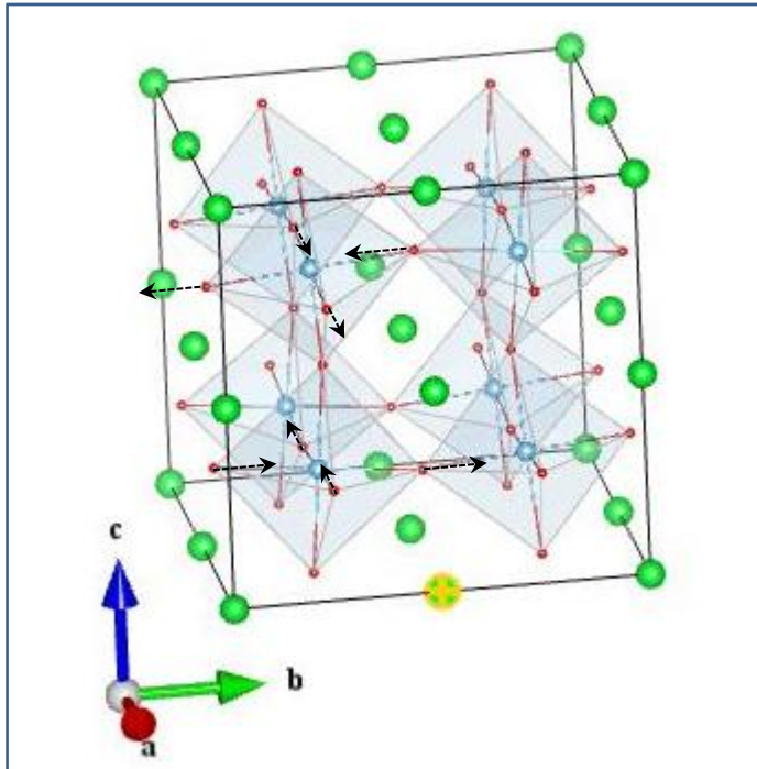
O1_B 1u (1)
