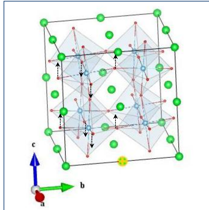
O1_B2u(1_2)
