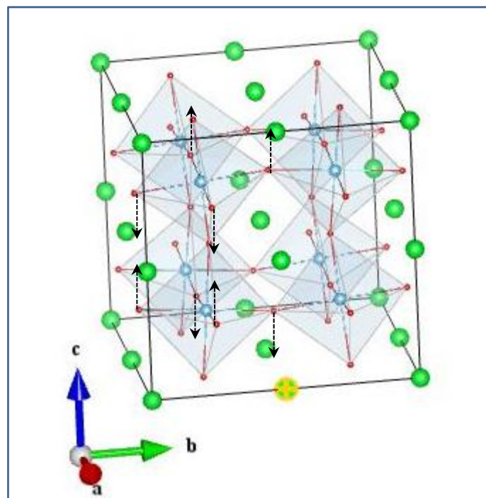
O1_A1g(1_2)
