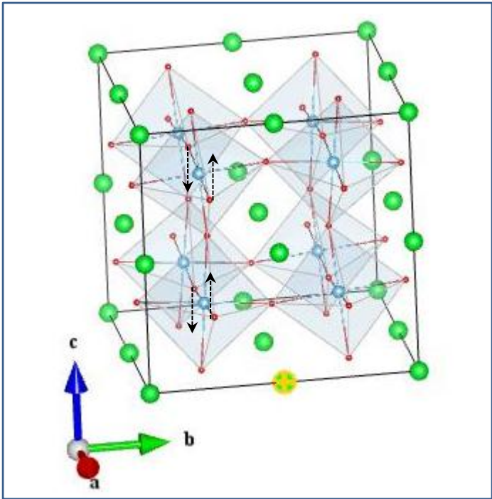
O1_Eg(3_1)
