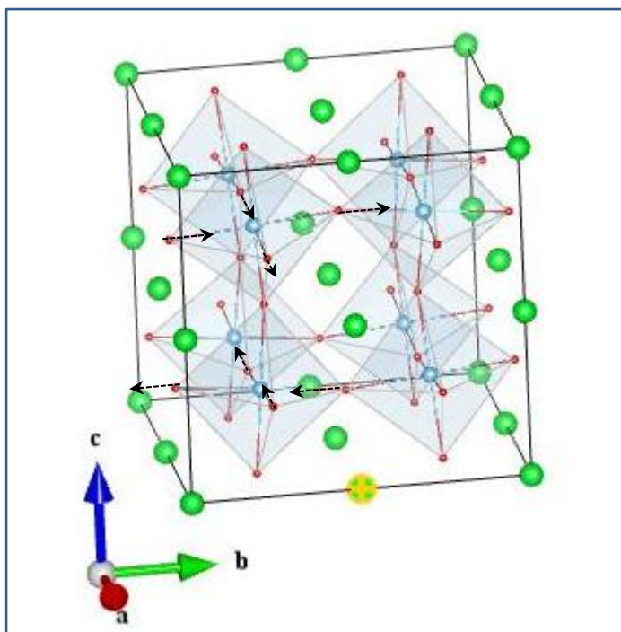
O1_A 1u (1)
