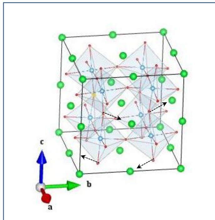
O2_A2g(1_1)
