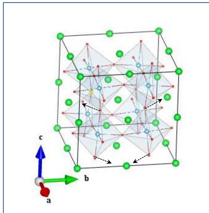
O2_B 1g (1_1)
