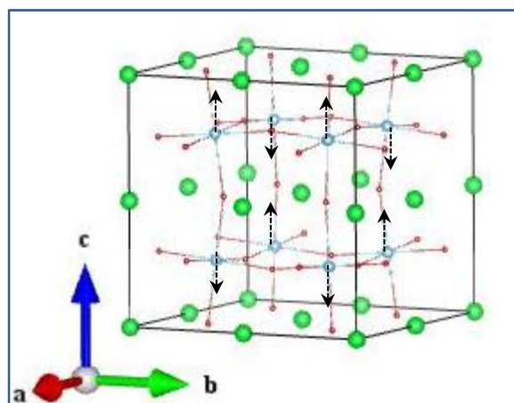
Ti_Eu (3_1)
