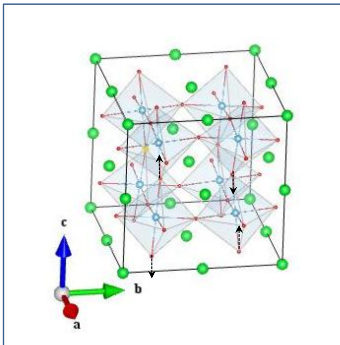
O2_Eg(1_1)
