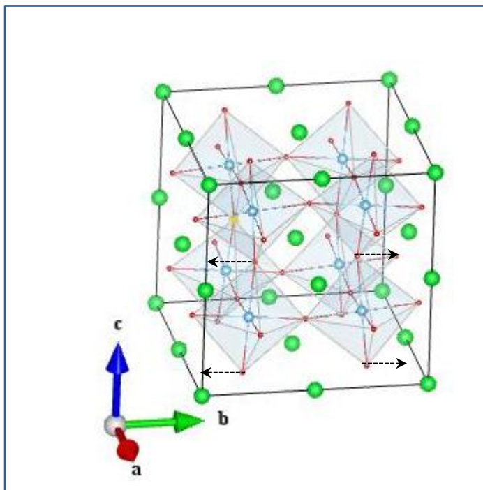
O2_Eu(1_1)
