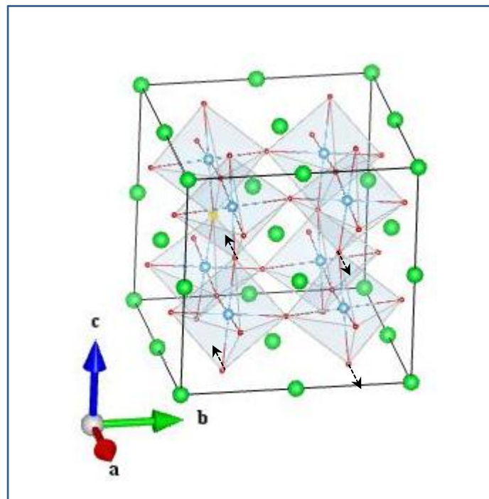
O2_Eu(1_2)
