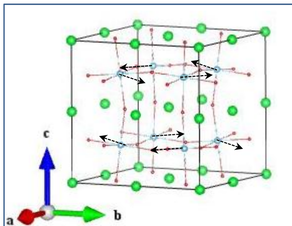
Ti_A 2u (1)
