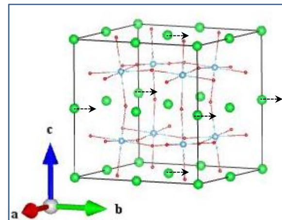
Sr 3 Eu (1_2)
