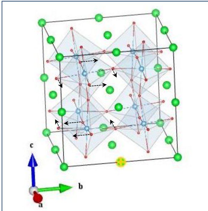
O1_B2u(1_1)
