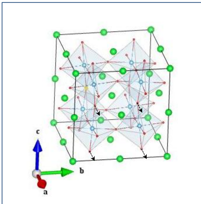
O2_Eu(2_1)
