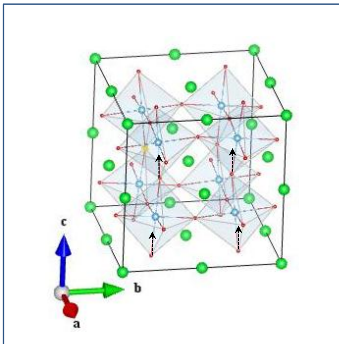
O2_A 2u (1)
