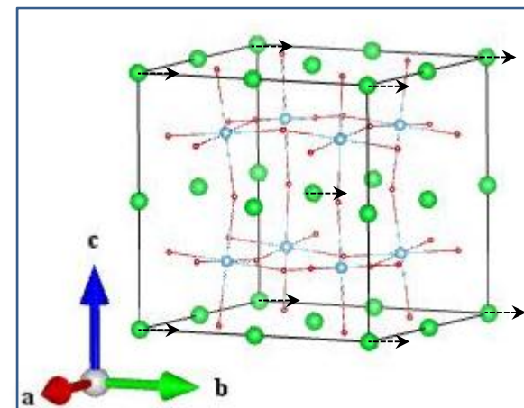
Sr 2 Eu (1_2)
