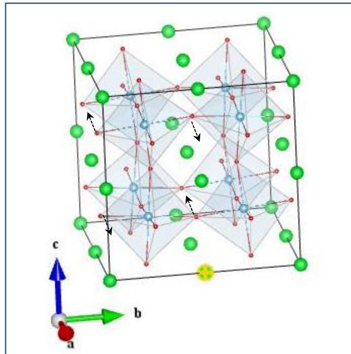
O1_Eg(1_2)
