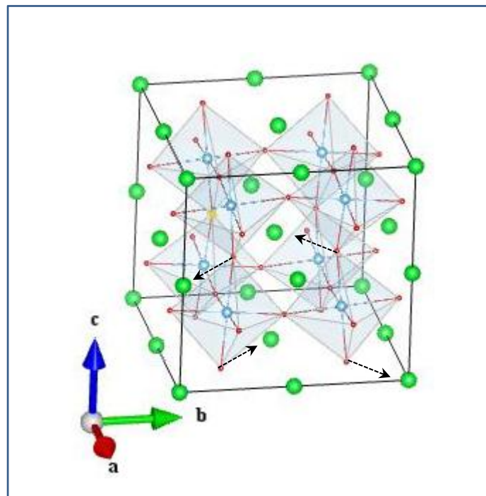
O2_B 2g (1)
