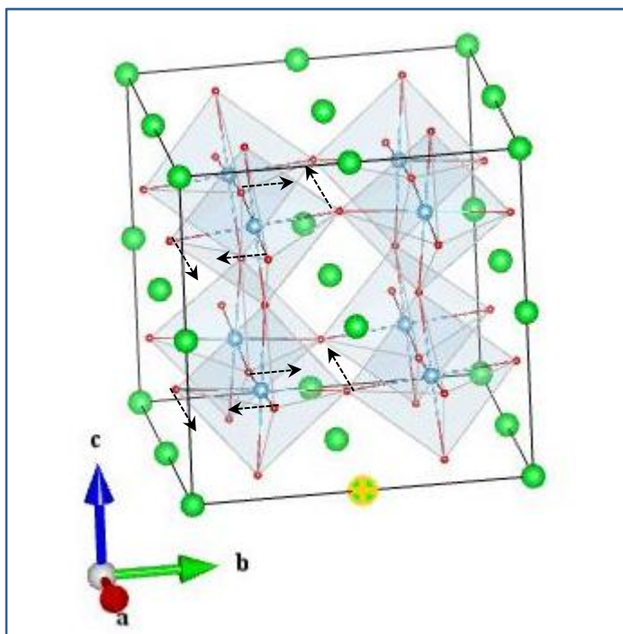
O1_A1g(1_1)
