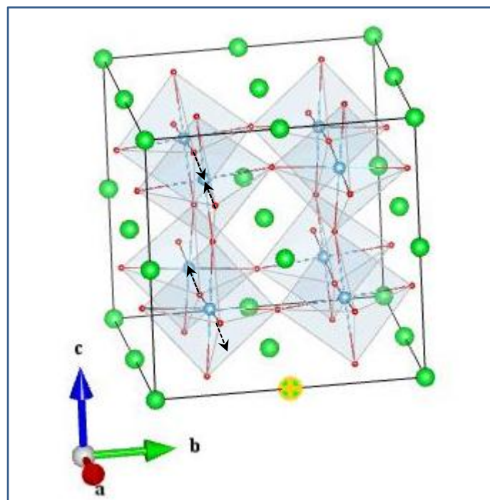
O1_Eg(2_2)
