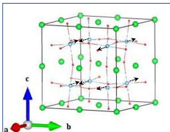
Ti_Eu (2_2)
