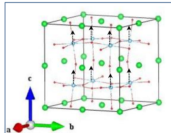
Ti_A 2u (1_2)
