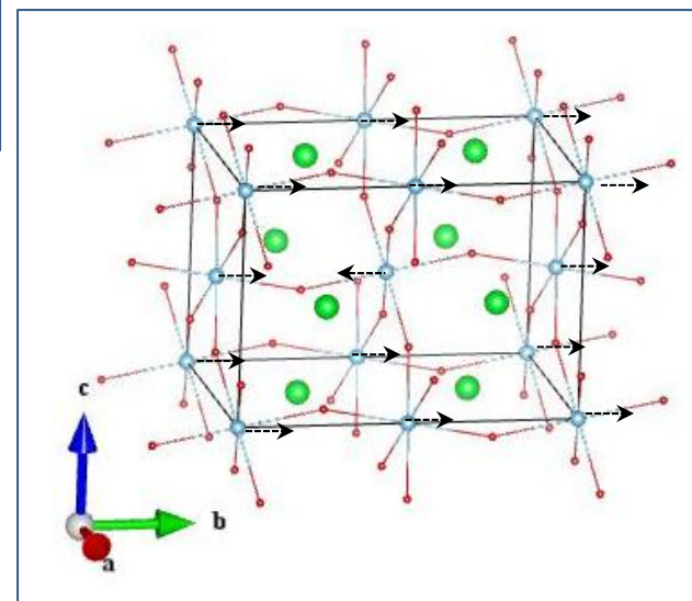
Ti_B 2u (1_2)
