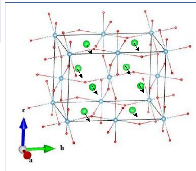
Sr_B 3u
