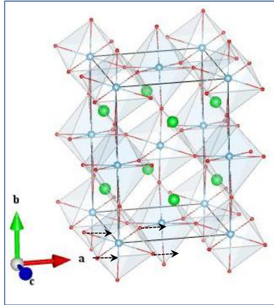
O1_B 3u (1_2)
