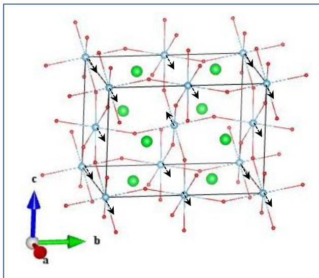
Ti_B 3u
