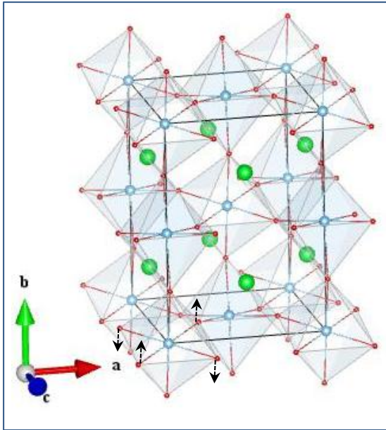
O1_B 3u (1_1)
