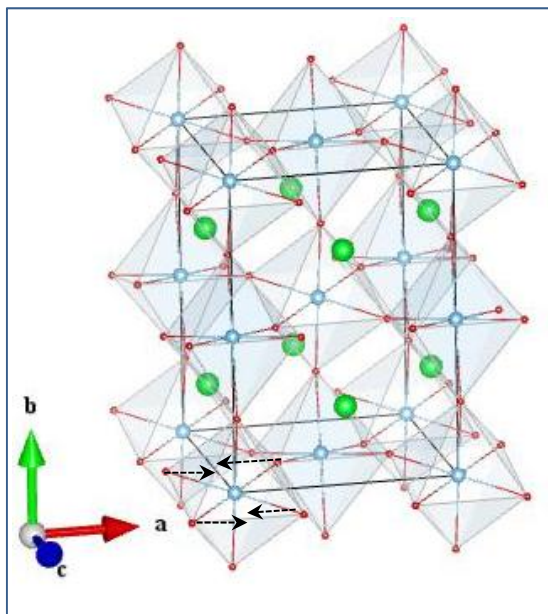
O1_B3g (1_1)
