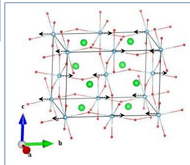
Ti_B 1u (1_2)
