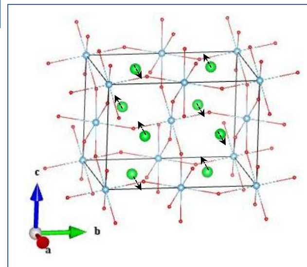
Sr_B2g
