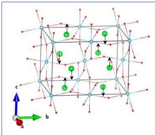
Sr_Ag
