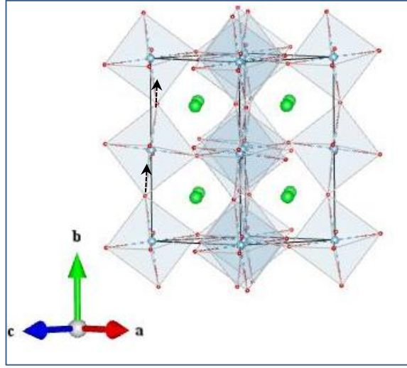
O2_B2u
