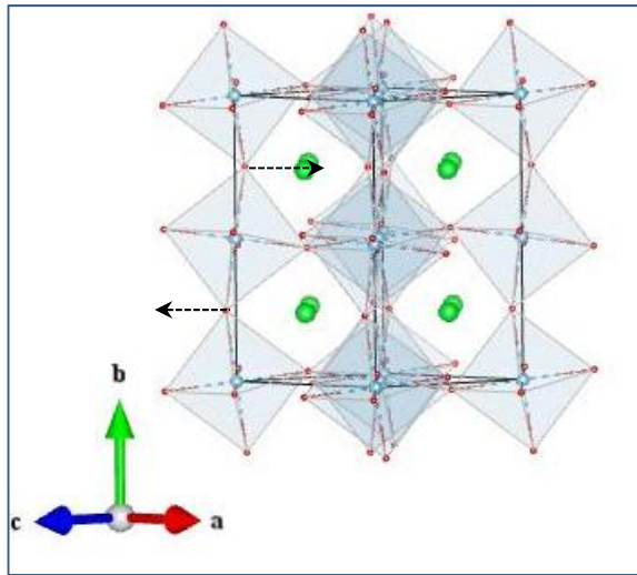
O2_B2g
