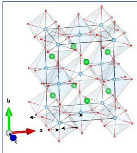
O1_B 1u (2)
