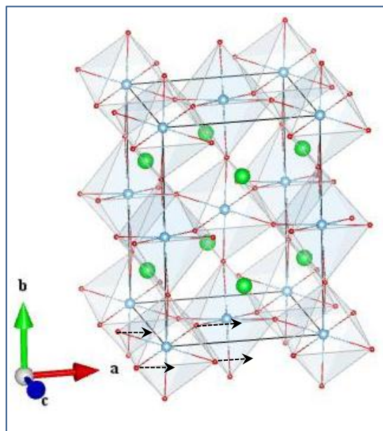
O1_B3g (1_2)
