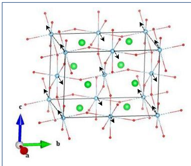
Ti_Au
