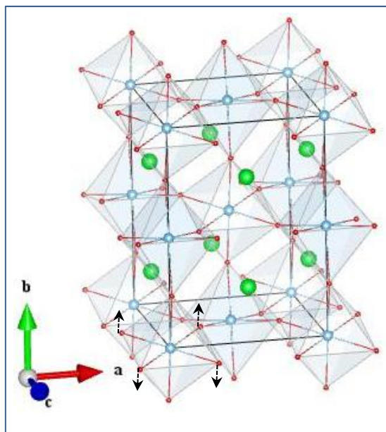
O1_B3g (1_1)
