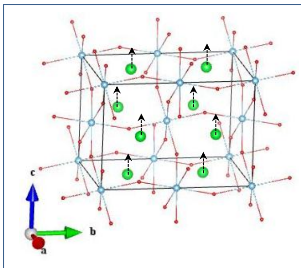
Sr_B1u
