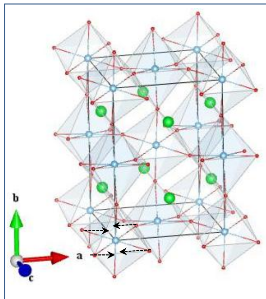
O1_B3g (1_2)
