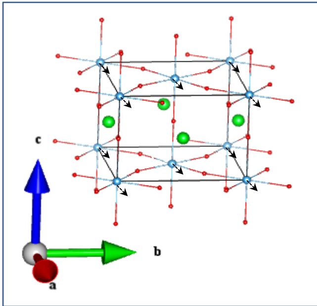
Ti_Eu (2_1)
