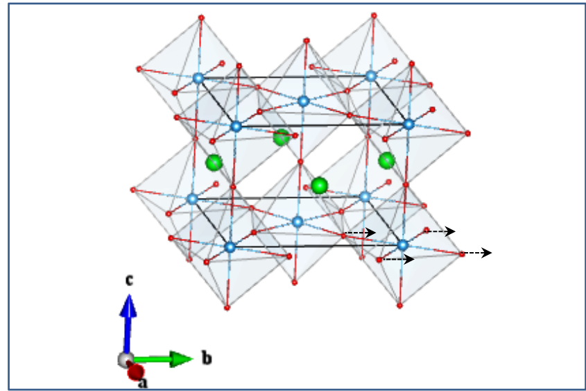
O2_Eu(2_2)
