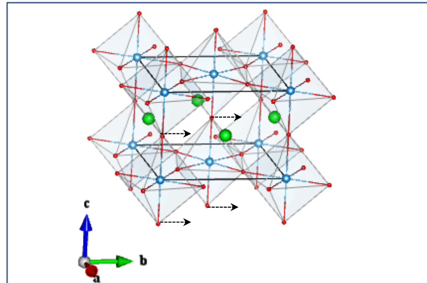
O1_Eu (2_1)
