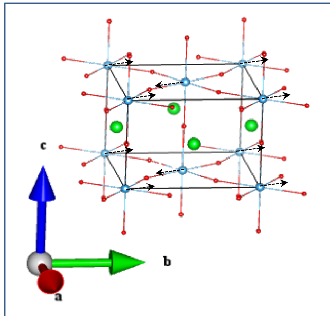
Ti_Eu (2_1)
