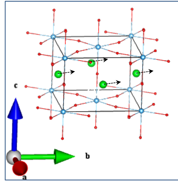
Sr_Eu (2_2)
