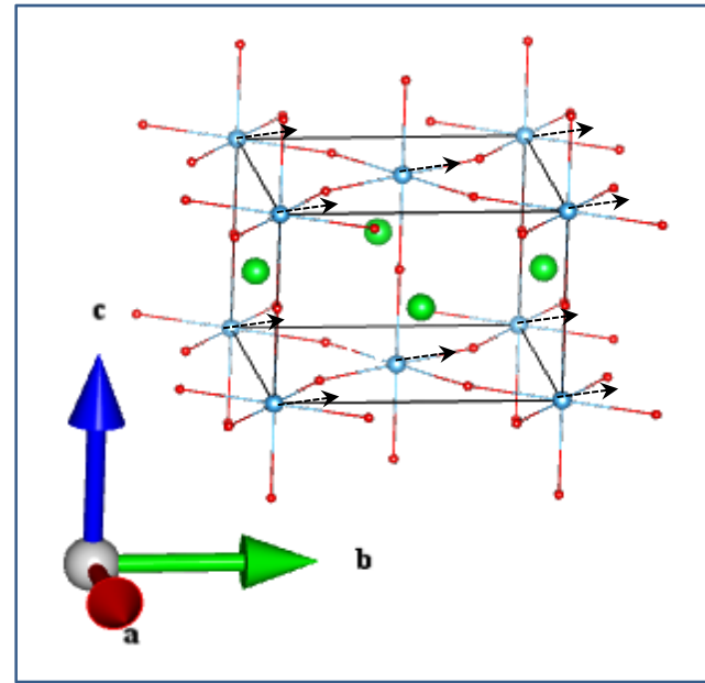
Ti_Eu (2_2)
