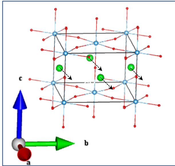
Sr_Eu (2_1)
