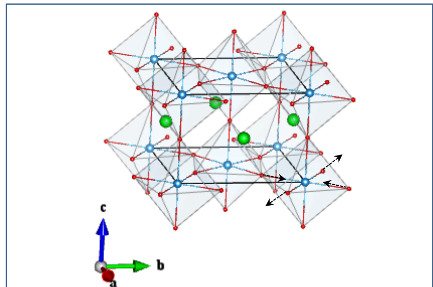
O2_B1g (1)
