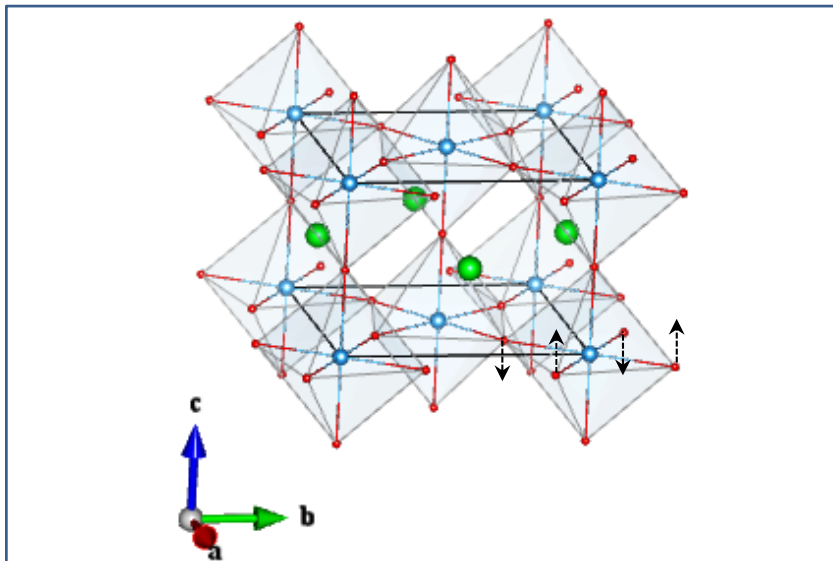
O2_E g (1_1)
