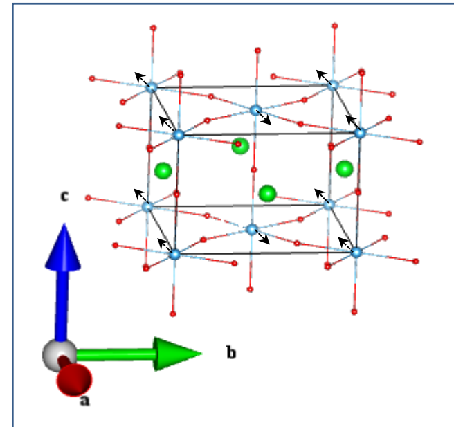
Ti_Eu (2_2)
