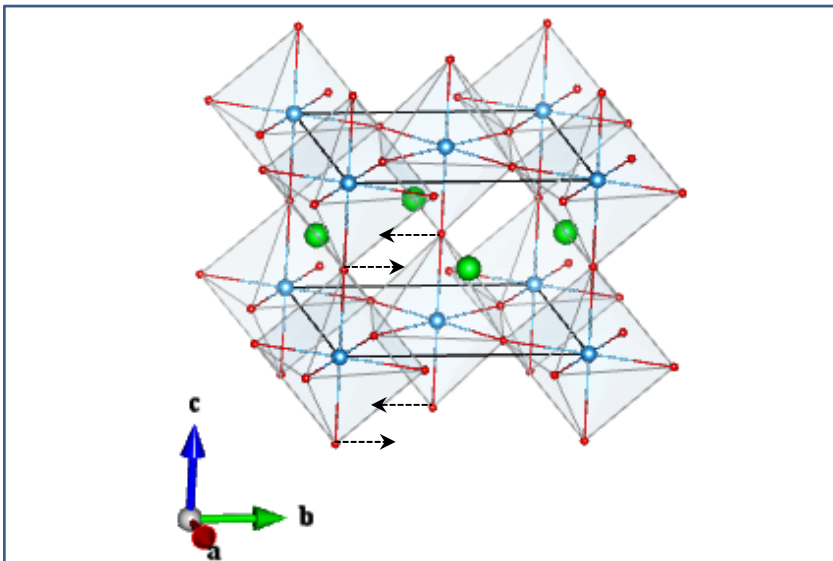
O1_Eu (2_1)
