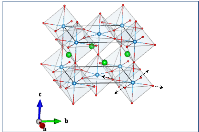
O2_B1g (1)
