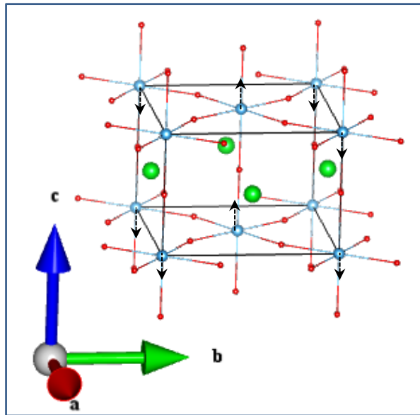
Ti_A 1u (1)
