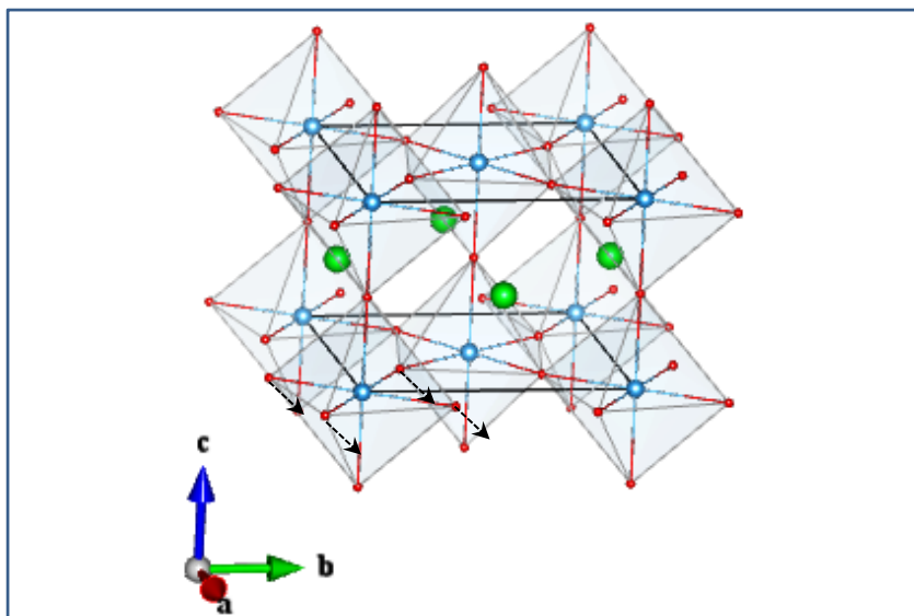
O2_Eu(2_1)
