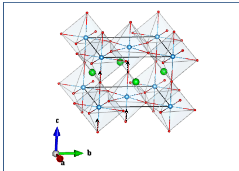
O1_A 2u (1)
