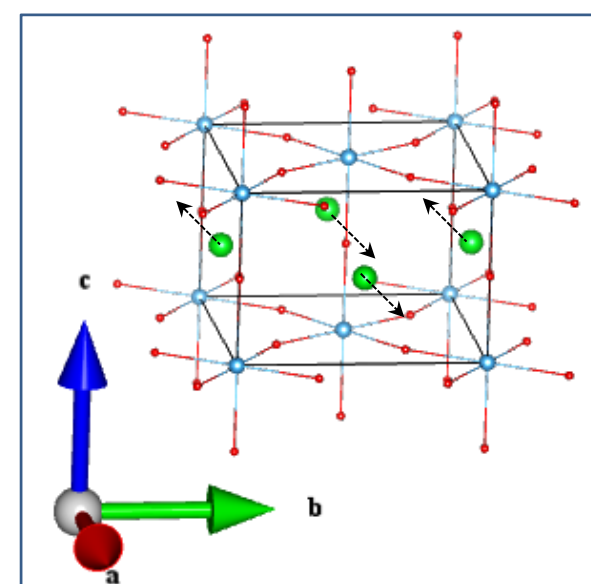
Sr_Eu (2_2)
