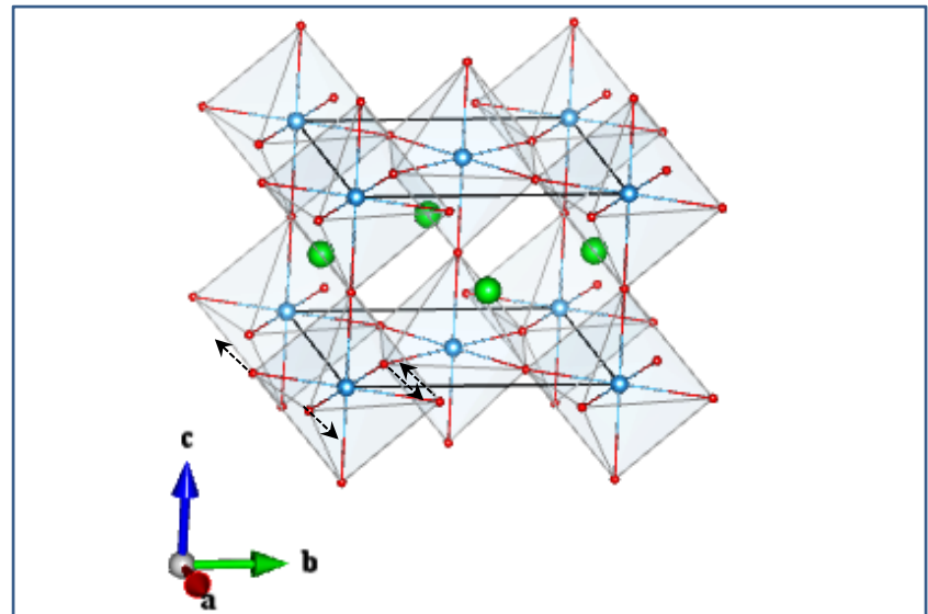
O2_Eu(2_2)
