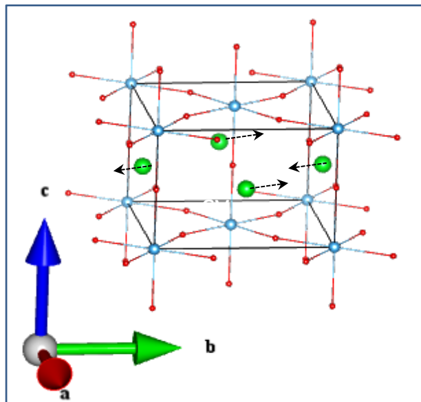
Sr_Eu (2_1)
