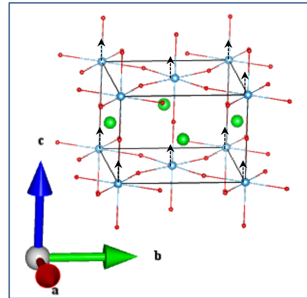
Ti_A 2u (1)
