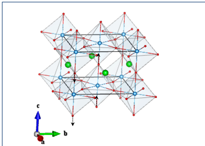
O1_A 1u (1)
