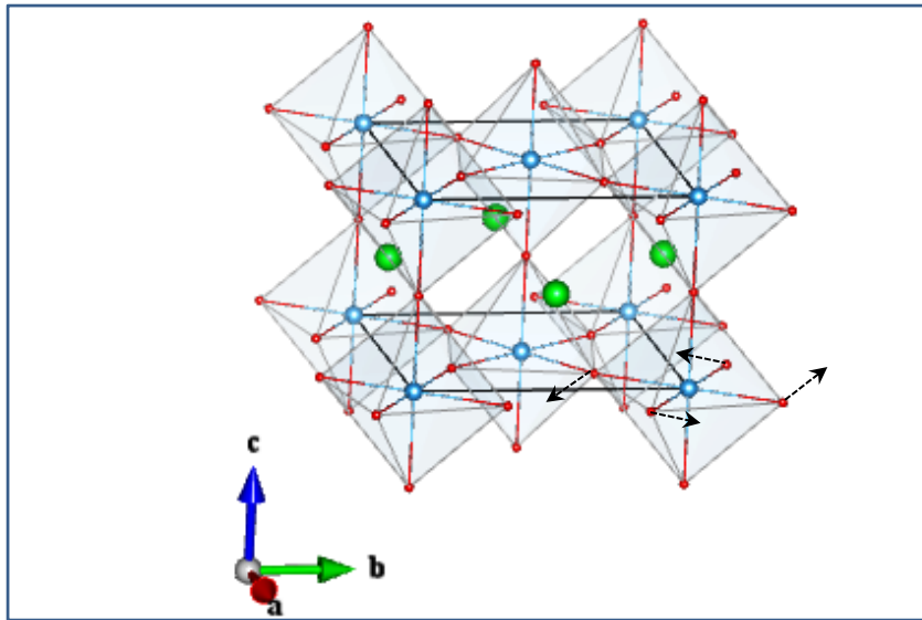
O2_A2u (1)
