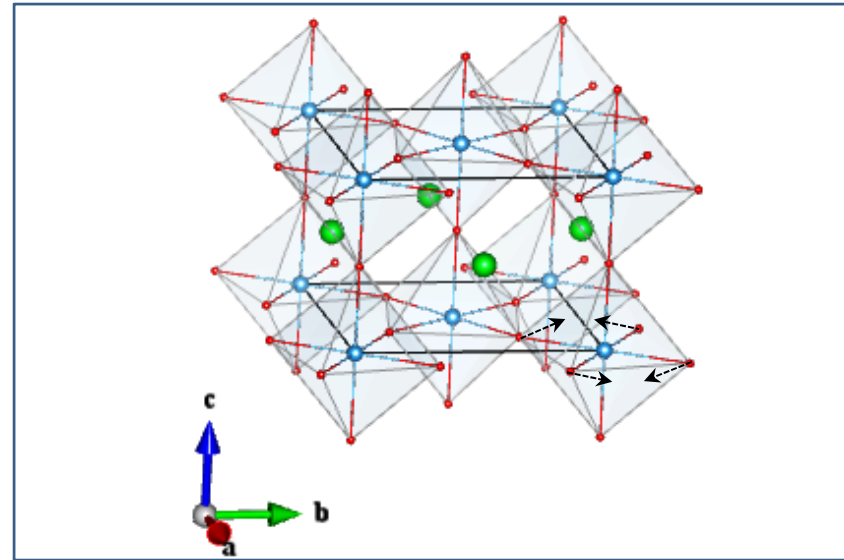
O2_E g (1_2)
