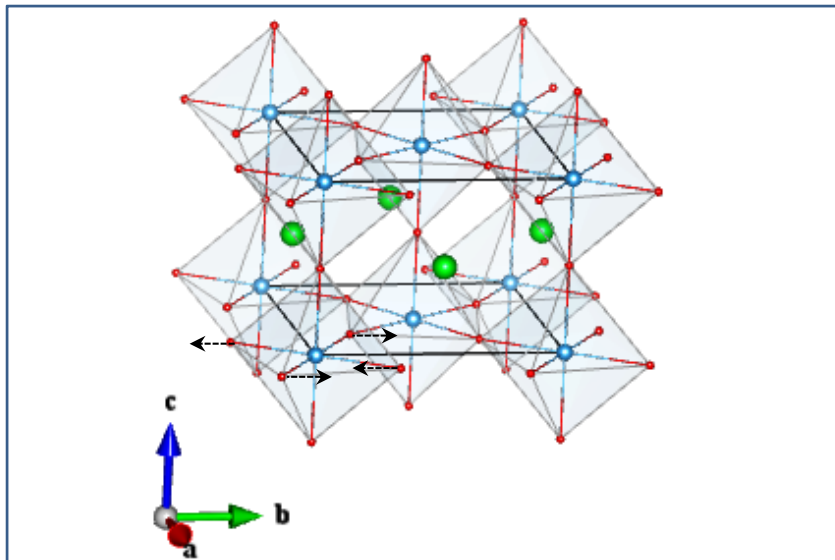
O2_Eu(2_1)
