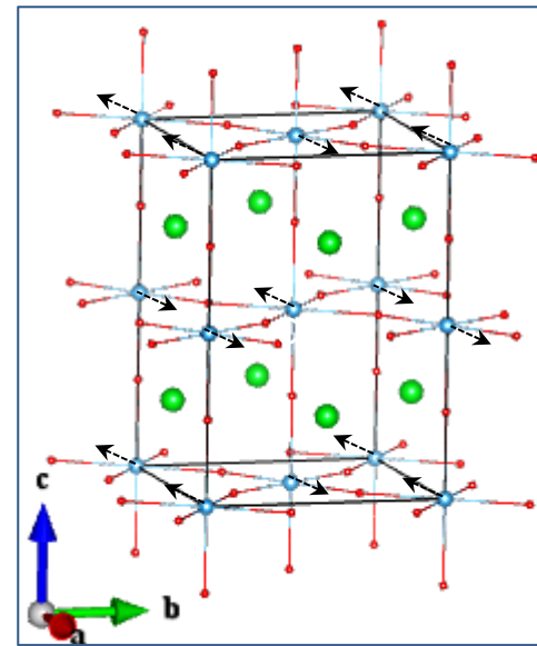
Ti_Eu_2_2
