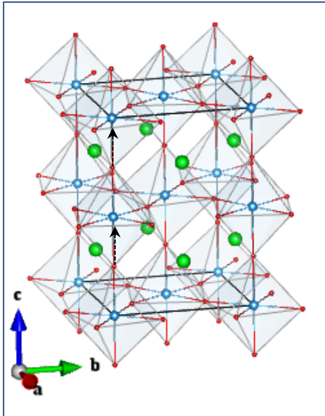
O2_E g (1_1)
