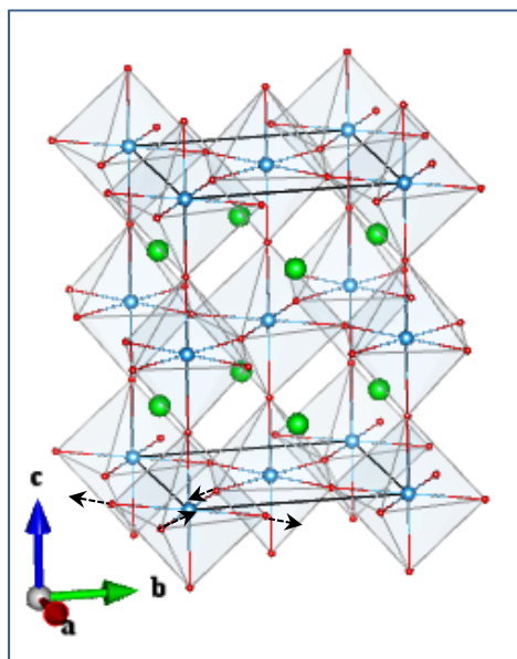
O1_B1g
