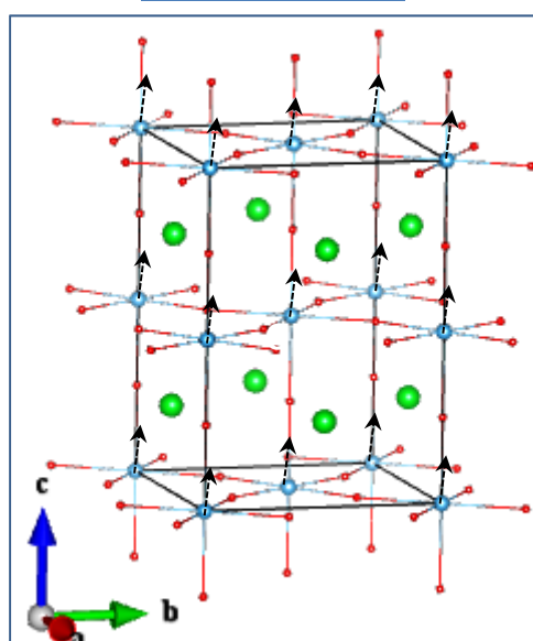
Ti_A2u
