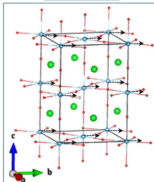
Ti_Eu_1_2
