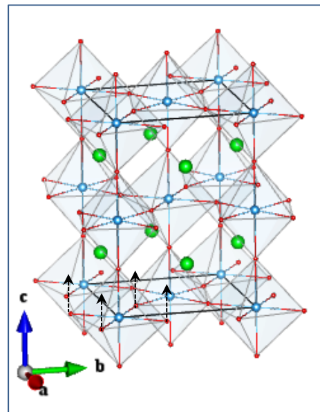
O1_A2u
