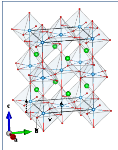
O1_B1u
