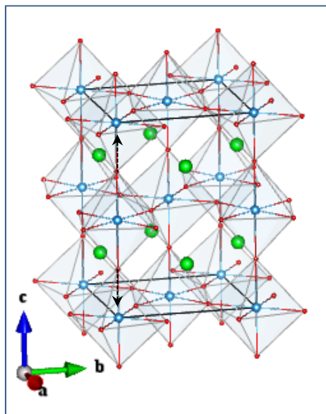
O2_E u (1_2)
