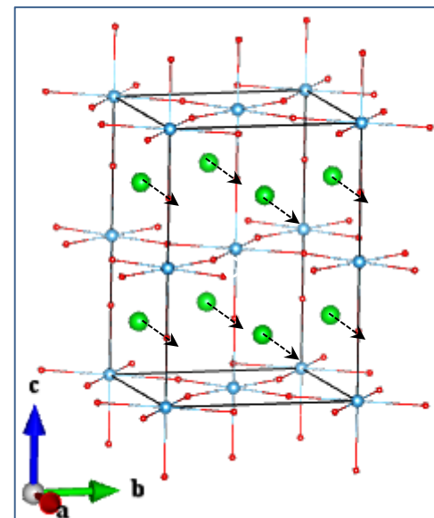
Sr_Eu 1
