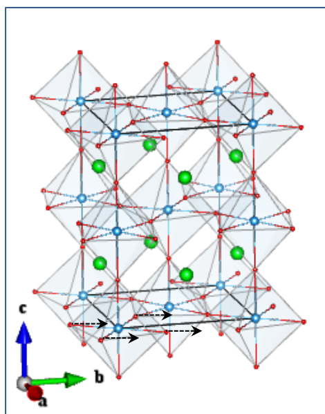
O1_Eu(2_2)
