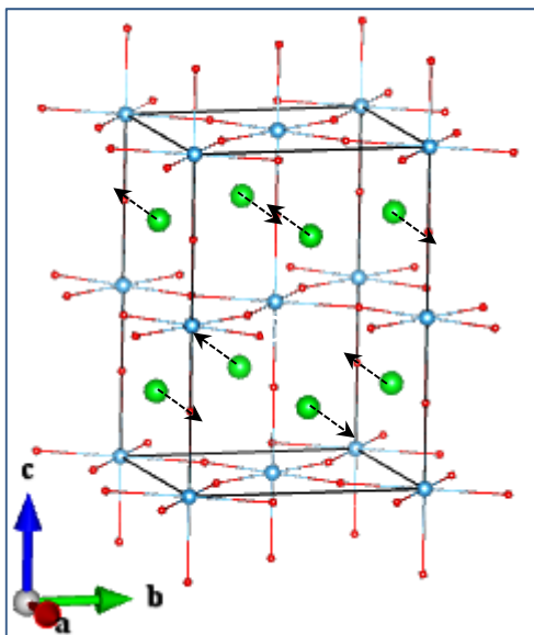
Sr_Eg 1
