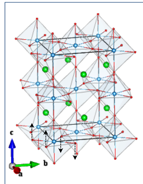
O1_Eg(1_2)
