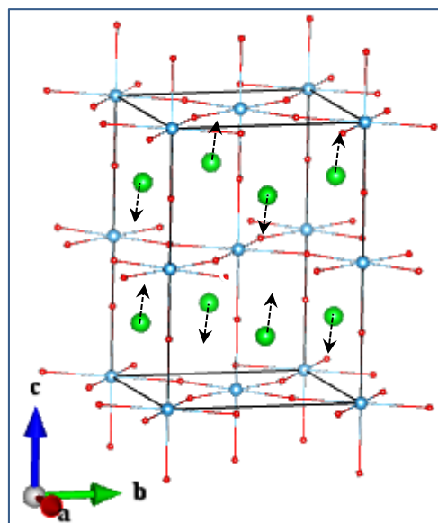
Sr_B 2g
