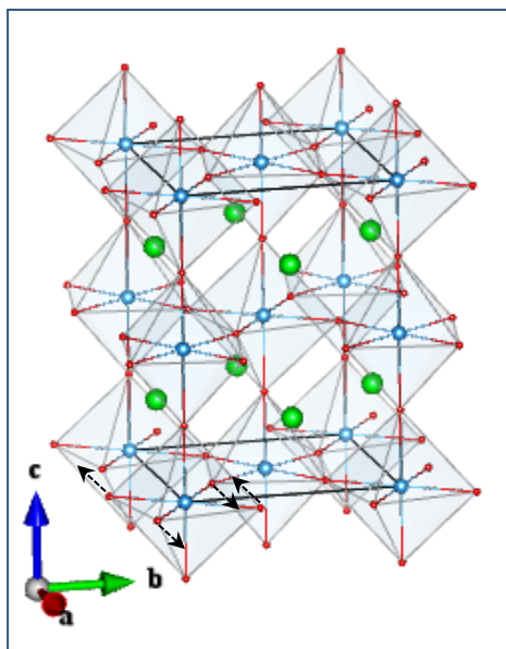
O1_Eg(1_1)
