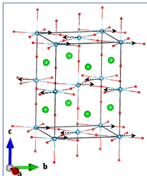
Ti_Eu_2_1
