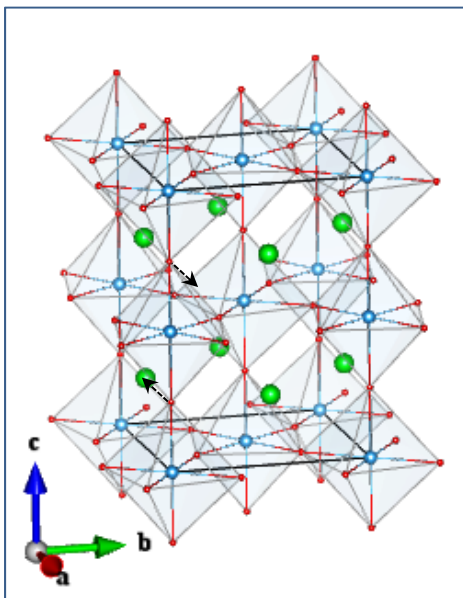
O2_E g (1_1)
