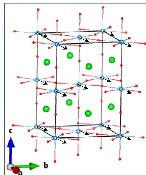
Ti_Eu_1_1
