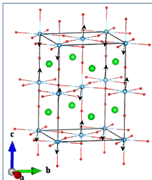
Ti_A1u
