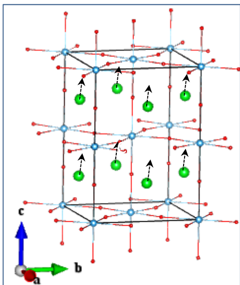
Sr_A 2u
