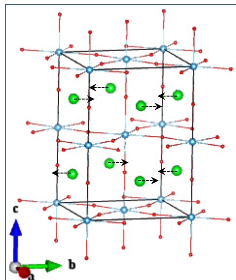
Sr_Eg 2
