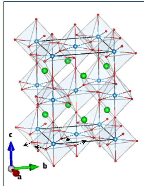
O1_B2g
