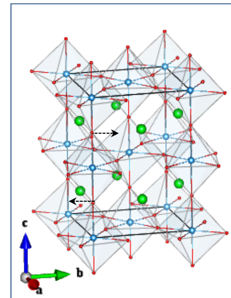
O2_E g (1_2)
