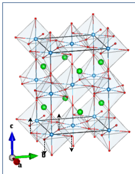
O1_Eg(1_1)
