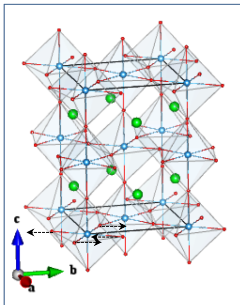
O1_Eu(2_2)
