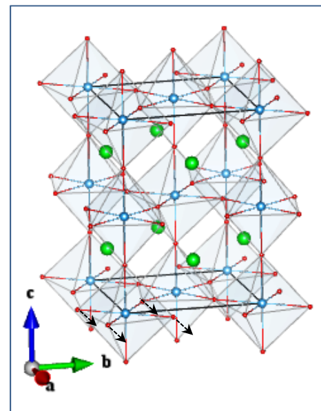
O1_Eg(1_2)
