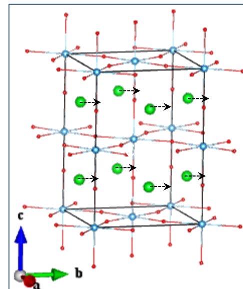
Sr_Eu 2
