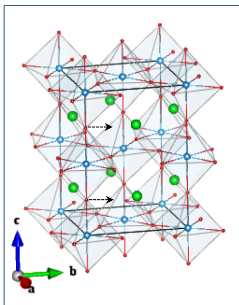
O2_E u (1_2)
