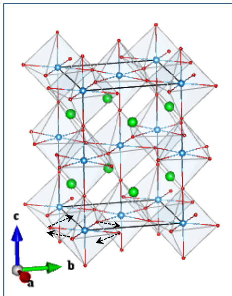
O1_A1g
