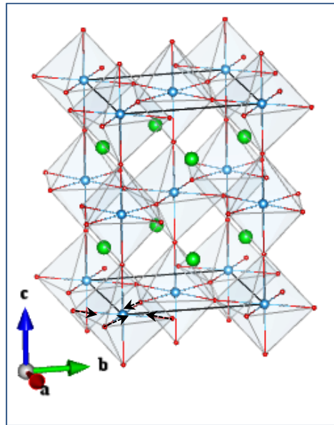
O1_A2g
