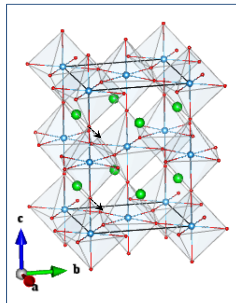
O2_E g (1_2)
